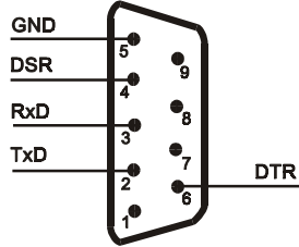
RS232c side
